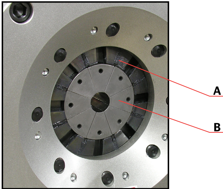
A) Master Die
